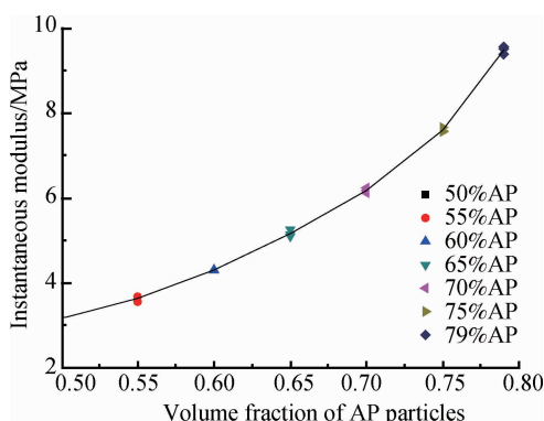
图 8 不同 AP 颗粒体积分数的复合固体推进剂瞬时模量
